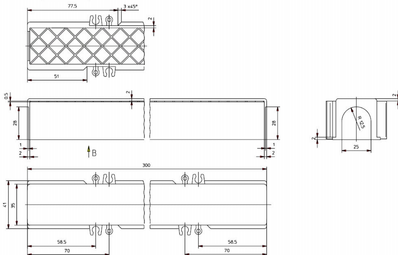
Teilansicht B:
